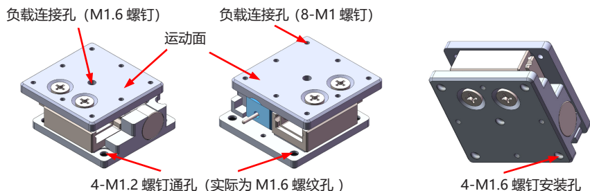
图 2 宏动台安装示意图
