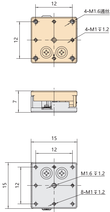
图 8 尺寸图
